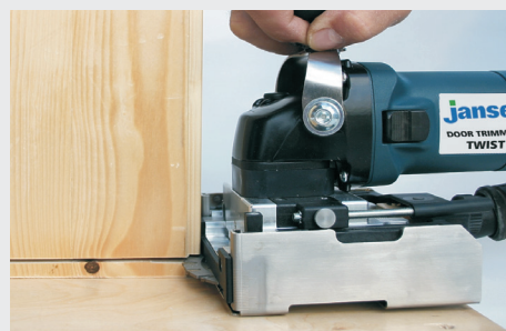
Podřezávání zárubní
